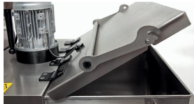
쉽게 멈추게 하는 경첩이 달린 탱크커버
